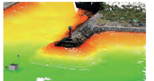
点群データ取得による水域施設の3次元化
