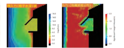
ブシネスク方程式モデルによる波浪変形計算
