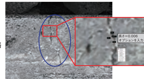
UAVによるオルソ画像の取得・損傷サイズの確認
