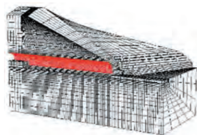
3次元トンネル掘進解析
