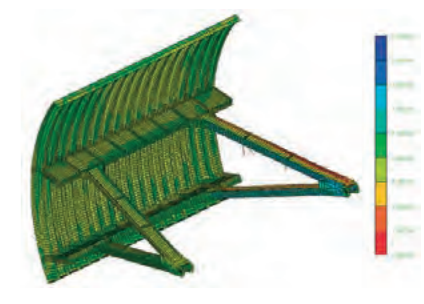
鋼構造物健全度解析(FEM解析)
