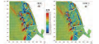
堆積侵食分布図および流れベクトル図
