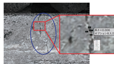
UAVによるORN画像の取得・損傷サイズの確認
