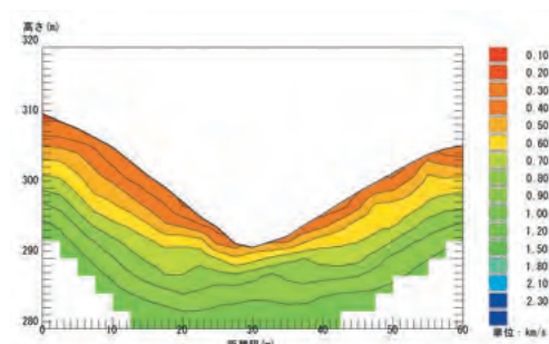
S波探査解析
