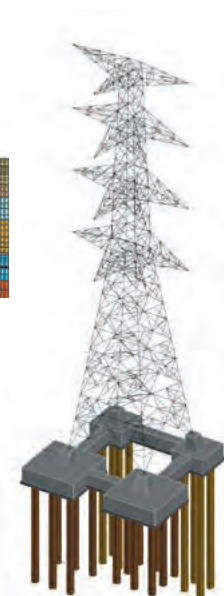
三次元構造解析
