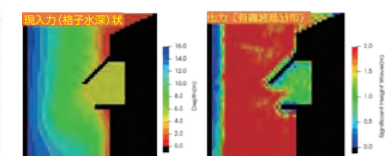
ビジネス方程式モデルによる波浪変形計算
