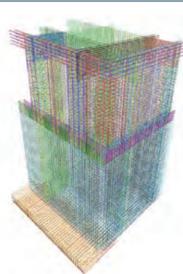
RCケーソン配筋図
