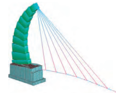
3次元動的解析
