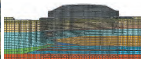
地盤変形解析
