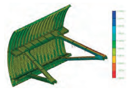
鋼構造物健全度解析（FEM解析）
