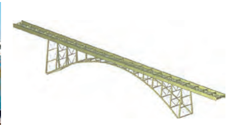
アーチ橋の耐震補強設計
