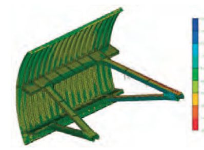
鋼構造物健全度解析 (FEM解析)
