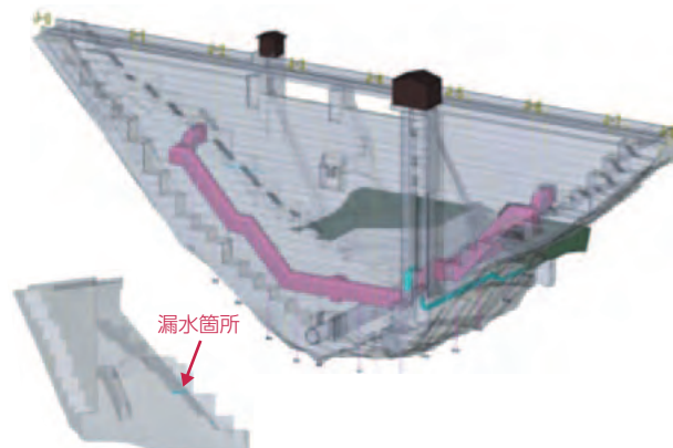
ダムの3次元モデル
