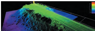
UAV+マルチビームによる三次元データ作成度調査
