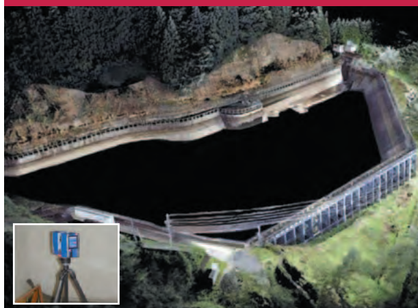
発電所の調整池の3次元モデル
